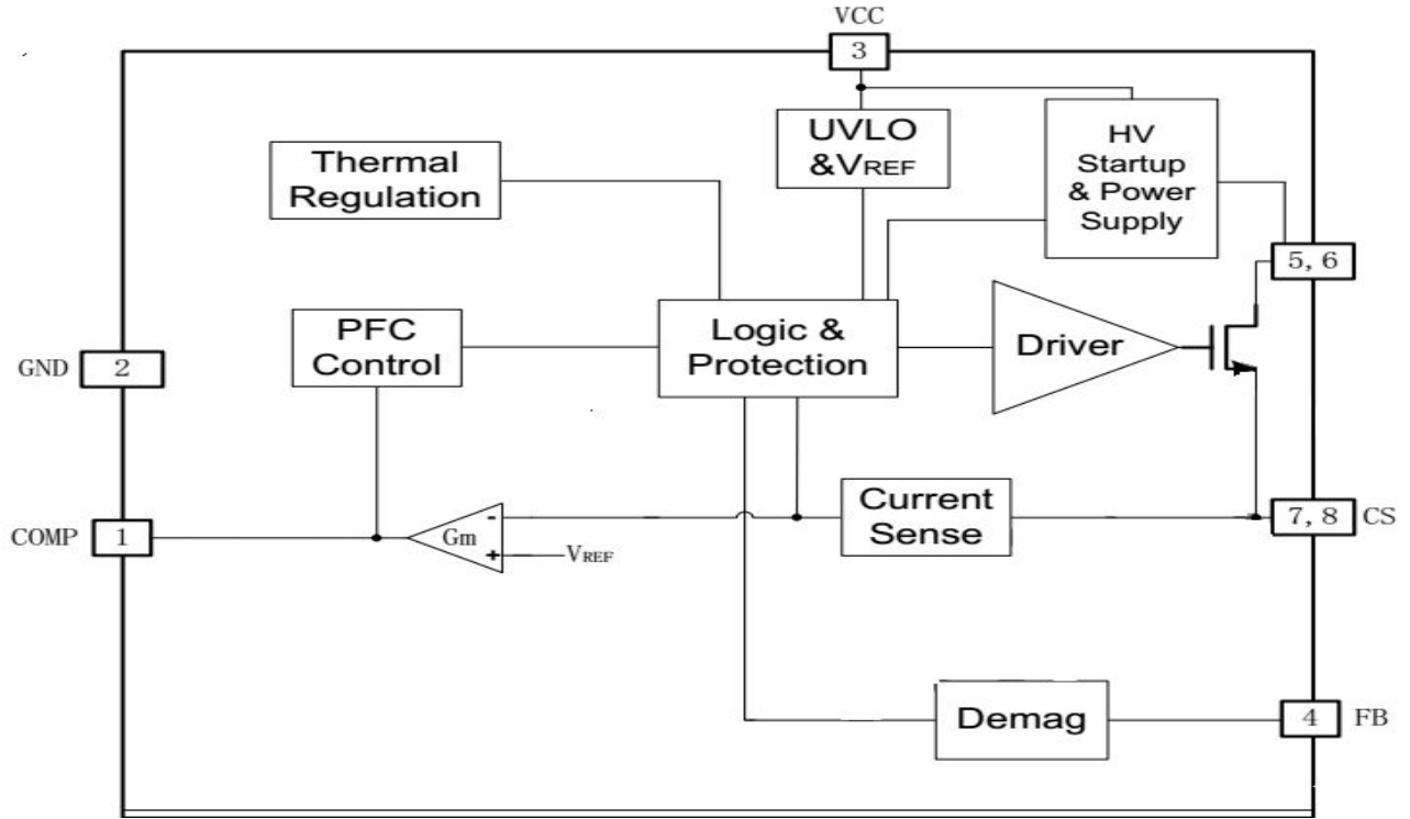
内部结构框图
