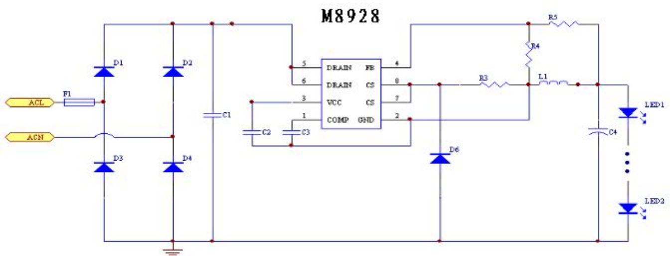
图1 M8928典型应用图
