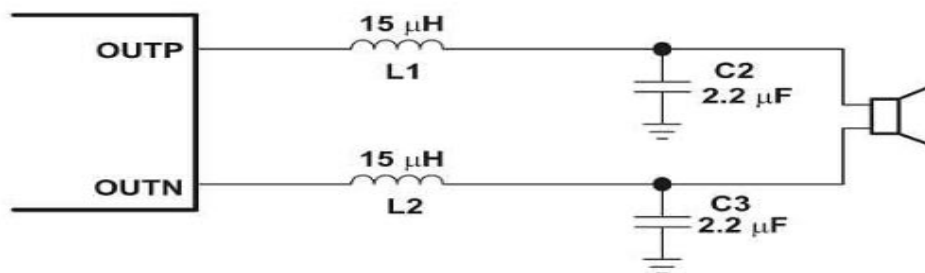
典型的扬声器负责为 4\Omega ，截止频率为 27\text{kHz} 的 LC 输出滤波器
