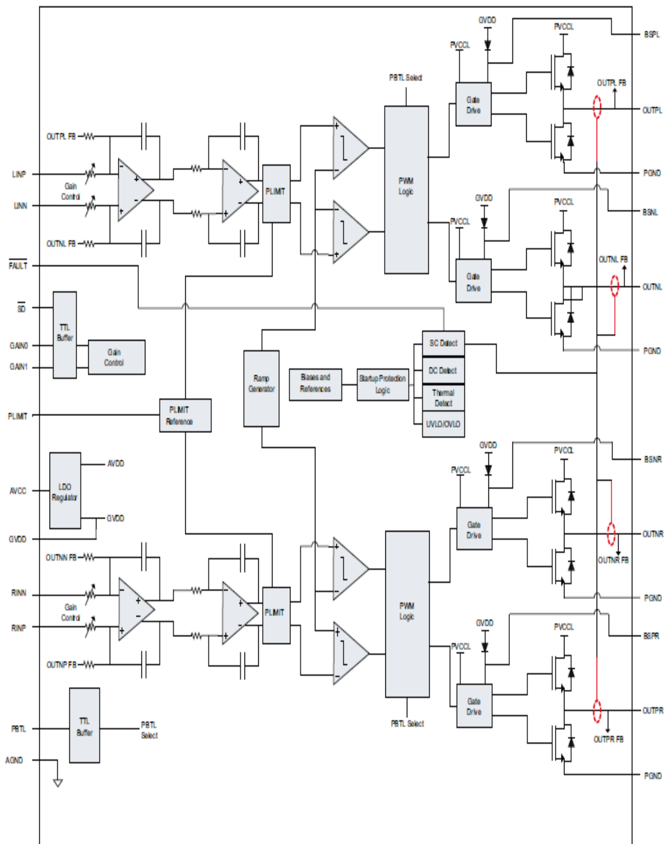
内部引脚图
