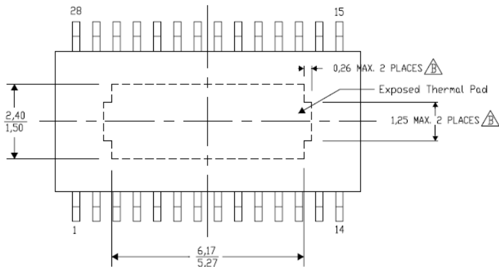
封装示意图 (HTSSOP) 28
